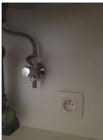
Aansluitingen vaatwasmachine
